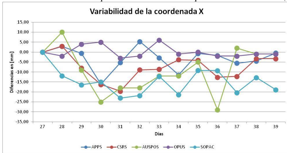
Variabilidad de los resultados del procesamiento en línea para las coordenadas (XYZ)
