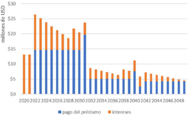
Ilustración 18 Reembolsos de préstamos y pagos de intereses, terminales combinados, millones de USD por año
