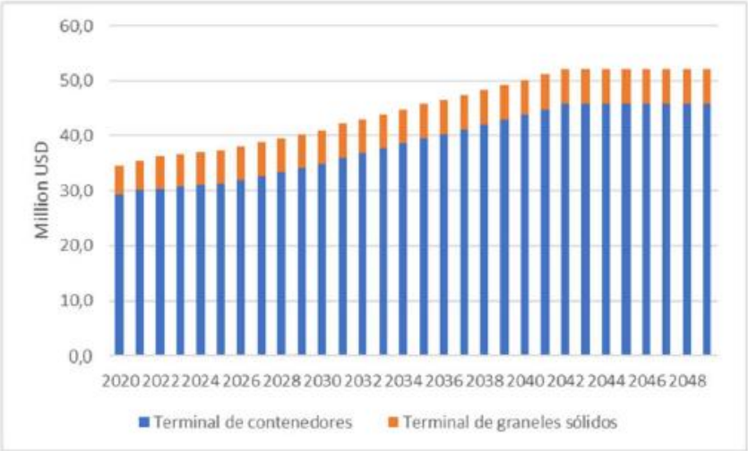
Ilustración 17 Costos operativos totales, terminales combinados, millones de USD por año
