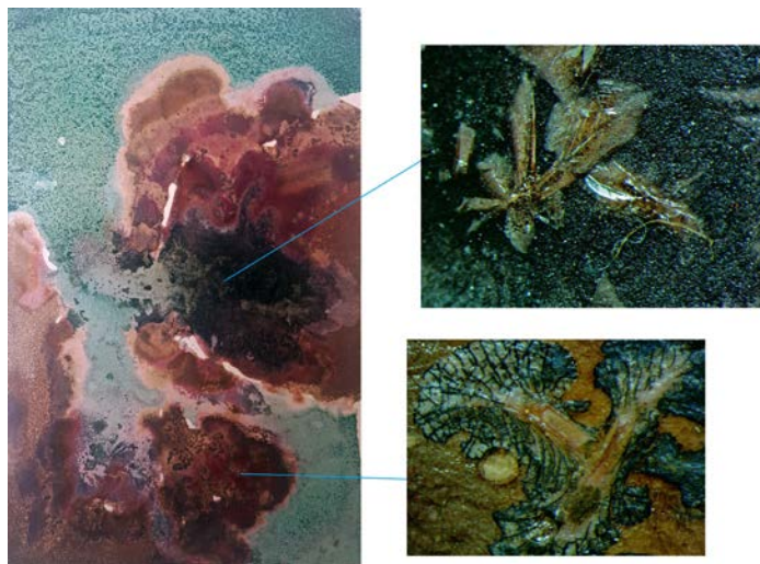
Figura 6. Muestra pictórica a partir de la mezcla de Co(CH_3COO)_2 y KCr(SO_4)_2 , adjunto de dos imágenes hechas con un microscopio estereoscópico.
