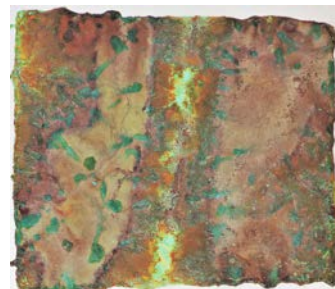
Figura 5. Proceso de cristalización de una aplicación pictórica de una mezcla de CuSO_4 y K_2Cr_2O_7 .
