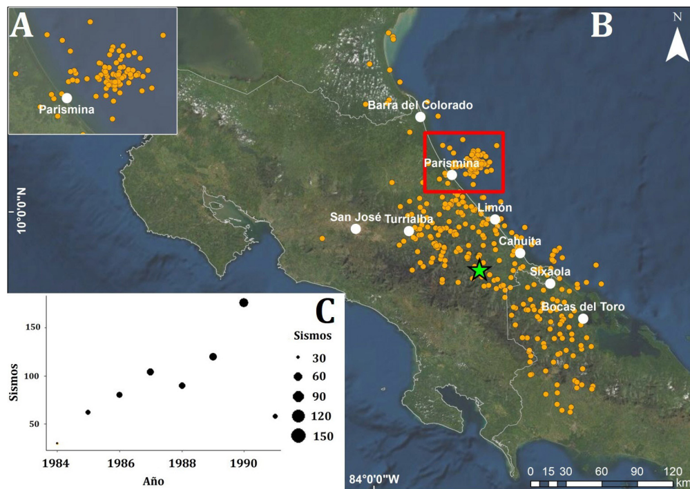
Fig. 5: A) Acercamiento de los epicentros relocados entre 1984 y el 22 de abril de 1991, cerca de Parismina. B) El epicentro del terremoto del Valle de La Estrella (Mw 7,6) se muestra con una estrella verde, los sismos se relocizaron usando cuatro o más estaciones sísmicas. C) comportamiento de la distribución temporal de la sismicidad entre 1984 y 1991, siendo 1990 el año con mayor actividad sísmica registrada.
