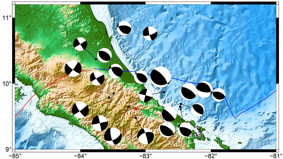
Fig. 9: Mecanismos focales desde 1988 hasta finales de setiembre del 2019; obtenidos del catálogo global GCMT (Dziewonski et al., 1981, Ekström et al., 2012) para la zona Caribe de Costa Rica y Panamá. Con una estrella de color roja se indica el epicentro del terremoto de Valle de La Estrella. Las líneas roja y azul indican los límites de placas CA-BP; con transición del tipo subducción (azul) a transcurrente (roja).
