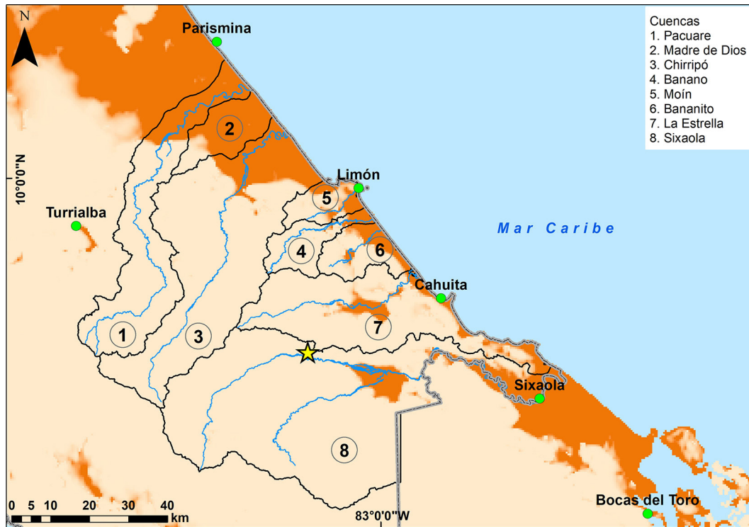
Fig. 13: Áreas afectadas por la licuefacción debido al terremoto del Valle de La Estrella, el modelo de licuefacción fue elaborado por Zhu et al. (2017) y facilitado por el Centro Nacional de Información sobre Terremotos del USGS (2020) ( https://earthquake.usgs.gov/earthquakes/eventpage/usp0004qpg/ground-failure/summary ), además se incluye la cartografía propuesta por Soulas (1991), la cual muestra una alta coincidencia al modelo de Zhu et al. (2017). La licuefacción se concentró en la costa y afectó ciudades como Limón en Costa Rica y Bocas del Toro en Panamá. El epicentro del terremoto se indica por una estrella amarilla y principales poblados por círculos verdes.
