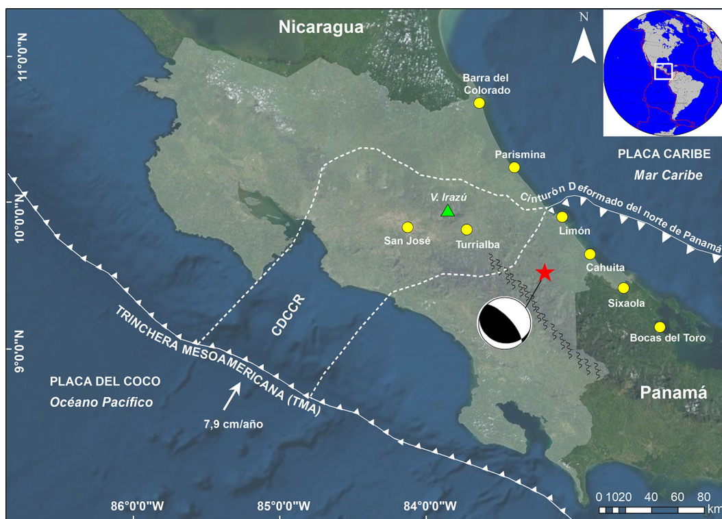
Fig. 1: Tectónica de Costa Rica, subducción de la placa del Coco bajo la placa Caribe y Bloque de Panamá a lo largo de la Trincherá Mesoamericana (TMA); el CDNP que es zona de pliegues y cabalgamiento en el Caribe de Panamá y Costa Rica (Climent et al., 2008) y el CDCCR que es límite W del Bloque de Panamá. El mecanismo focal del terremoto del Valle de la Estrella de 1991 (GCMT, 2020) es mostrado en la figura; con strike/dip/rake de 103°/25°/58° y el epicentro relocalizado en este trabajo se indica por una estrella roja; por círculos amarillos se indican las principales localidades afectadas por el terremoto de 1991, por un triángulo verde el macizo del volcán Irazú y la cordillera de Talamanca por líneas negras. Se indica la velocidad relativa de convergencia CO-CA 7,9 cm/año de acuerdo con el modelo GSRM2.1 (Kreemer et al., 2014), calculada usando la calculadora de movimiento de placas de UNAVCO ( https://www.unavco.org/software/geodetic-utilities/plate-motion-calculator/plate-motion-calculator.html ).
