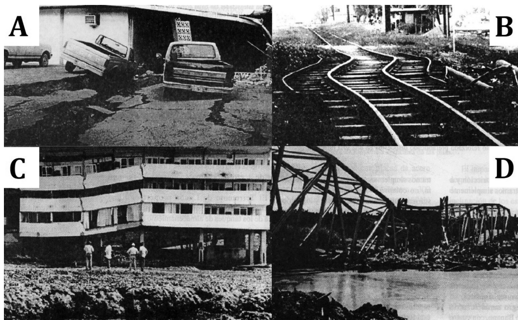
Fig. 14: Principales efectos de la licuefacción en Costa Rica y Panamá: A) Grietas en las oficinas de la Chiriquí Land Company en Changuinola debido a desplazamientos laterales. B) Daños en el puente del ferrocarril en Changuinola, Panamá, debido a desplazamientos laterales. C) Hotel Las Olas en la ciudad de Limón, parcialmente colapsado, sus bases fueron construidas sobre material coralino. D) Puente sobre el río La Estrella colapsado debido a la falta de mecanismos de soporte para mitigar los desplazamientos laterales. Las imágenes A y B fueron tomadas de Camacho y Viquez (1994) y las imágenes C y D de Sauter (1994).
